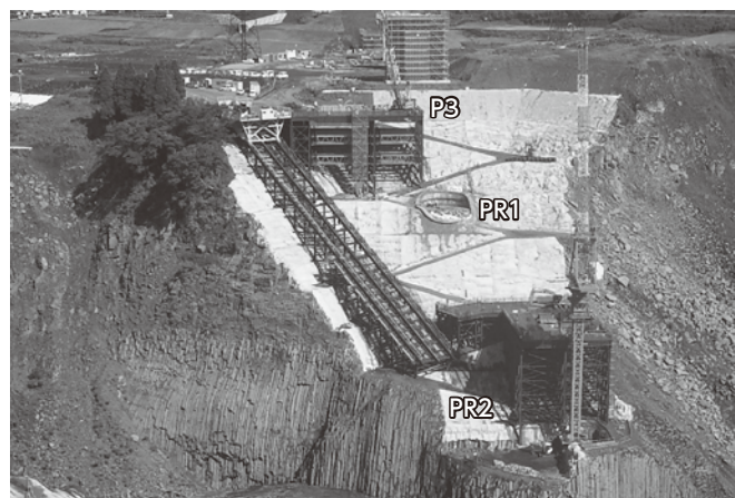
阿蘇大橋の下部工 (基礎工) 工事をしています。
