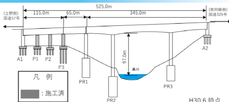
阿蘇大橋 (立野) 側 (撮影日：平成30年6月22日)
