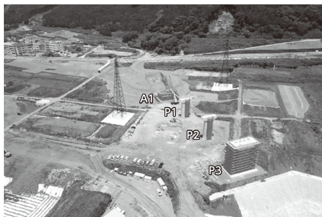
阿蘇大橋の下部工 (A1) 工事をしています。
