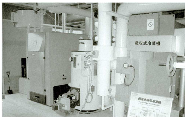
ペレットボイラシステム一式
